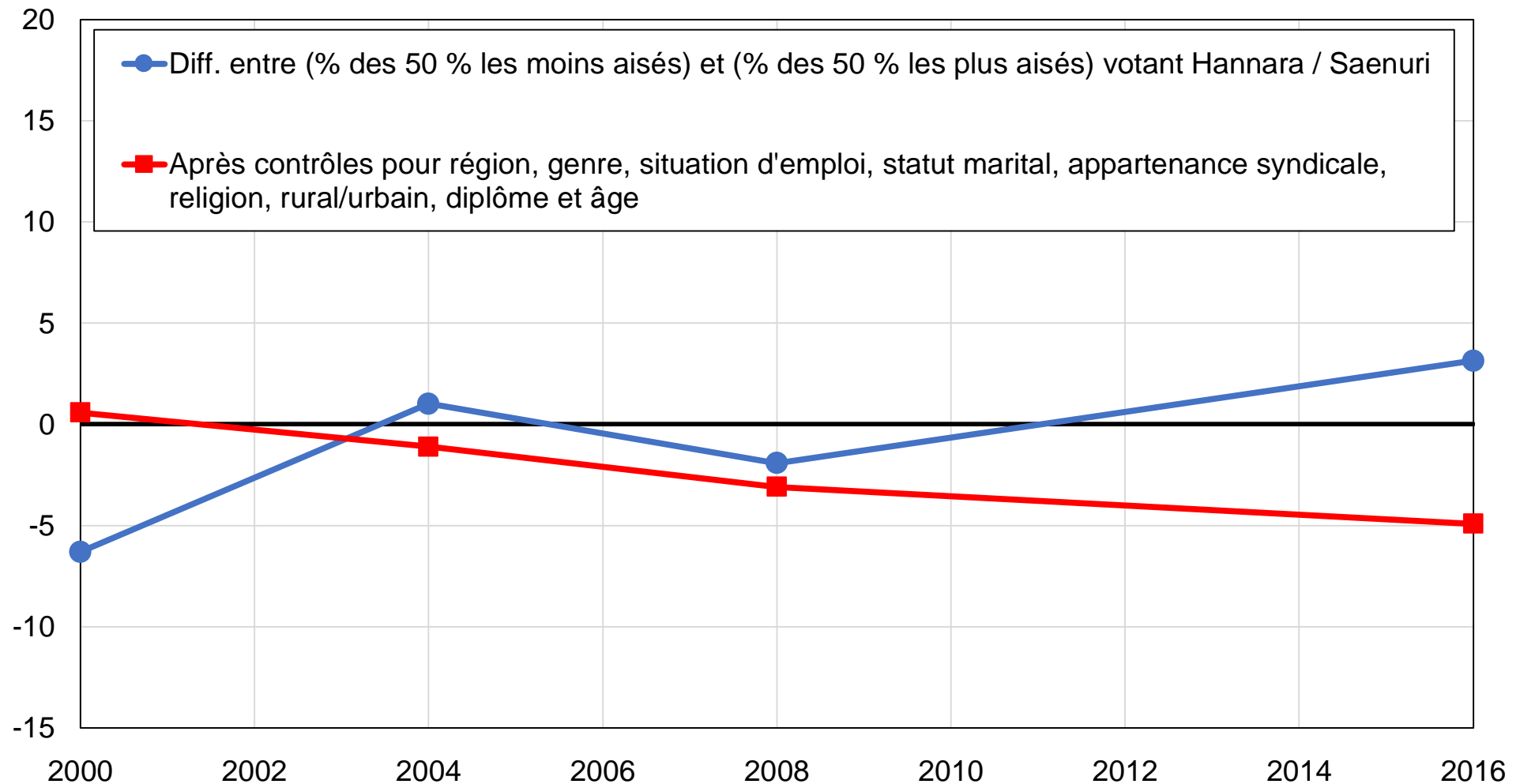
Graphique 13.5 - Vote et revenu en Corée du Sud, 2000-2016
