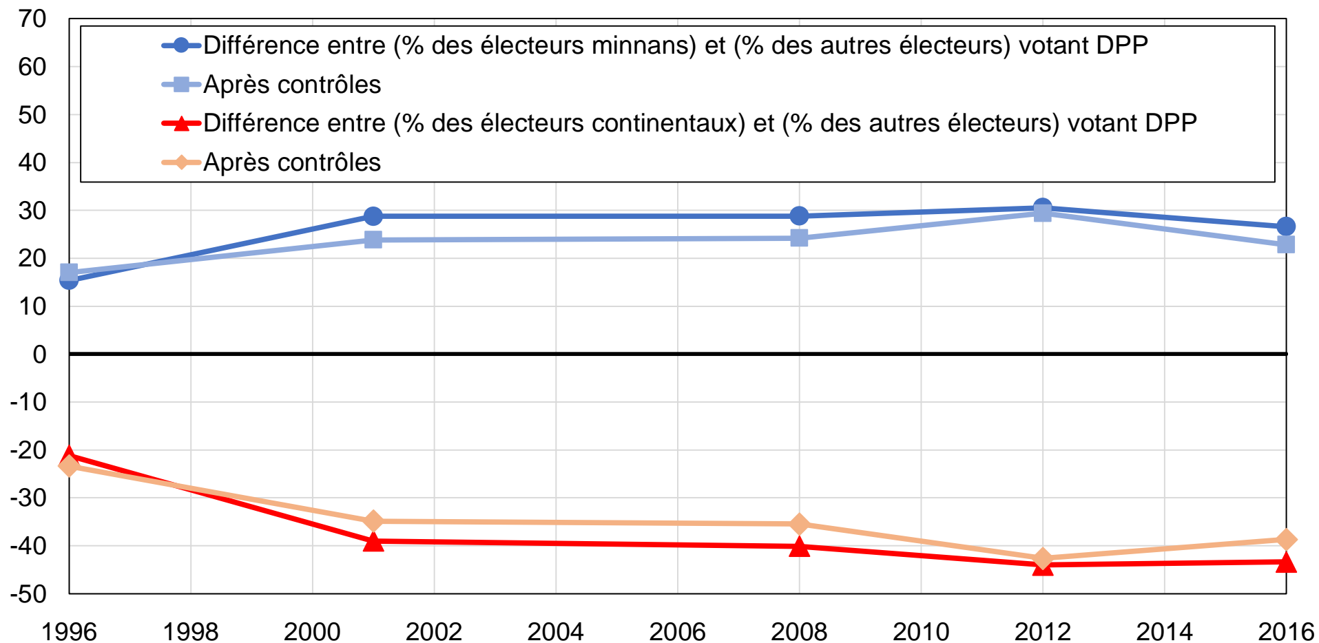
Graphique 13.8 - Le clivage ethnique à Taïwan, 1996-2016
