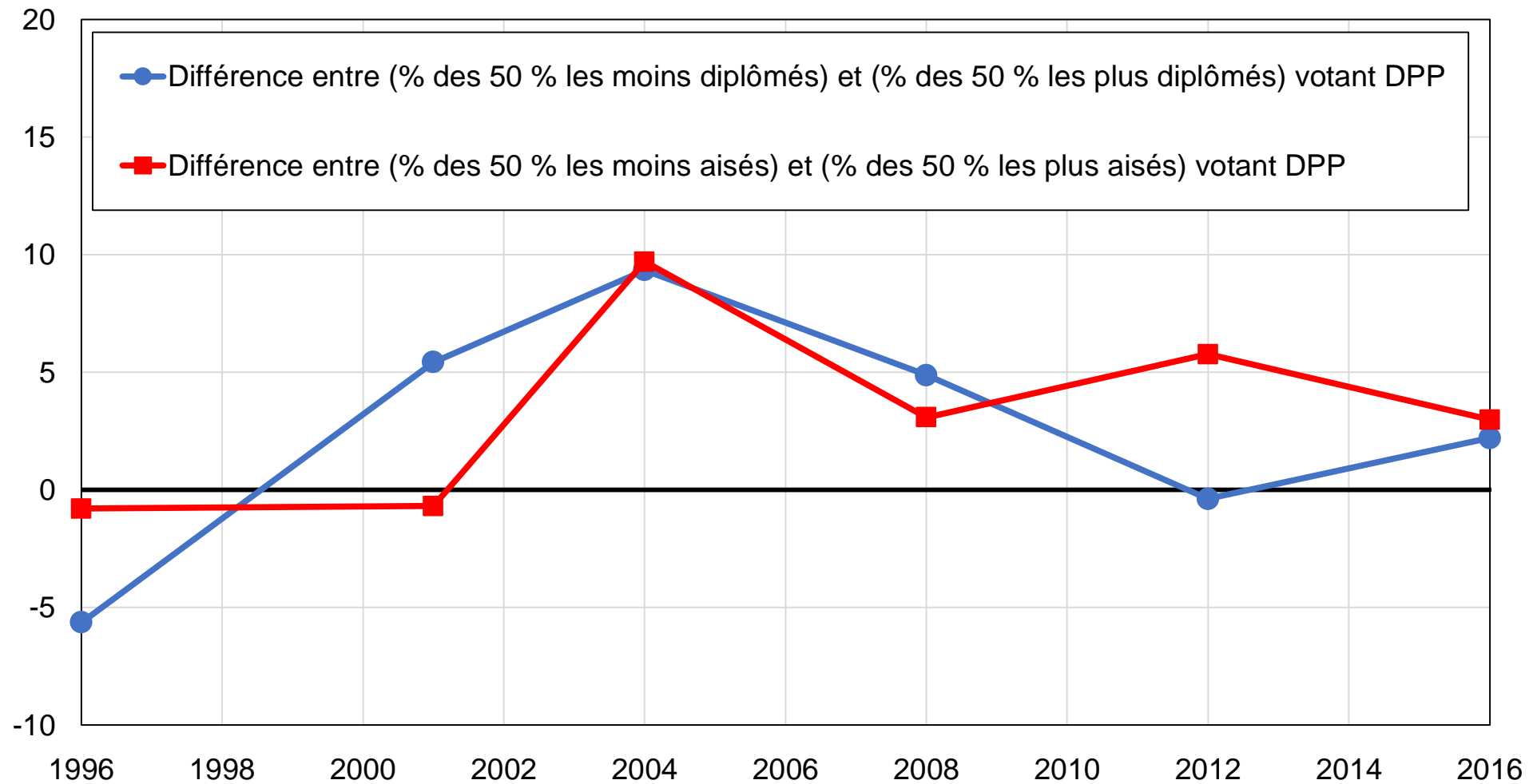
Graphique 13.10 - Vote, revenu et diplôme à Taïwan, 1996-2016
