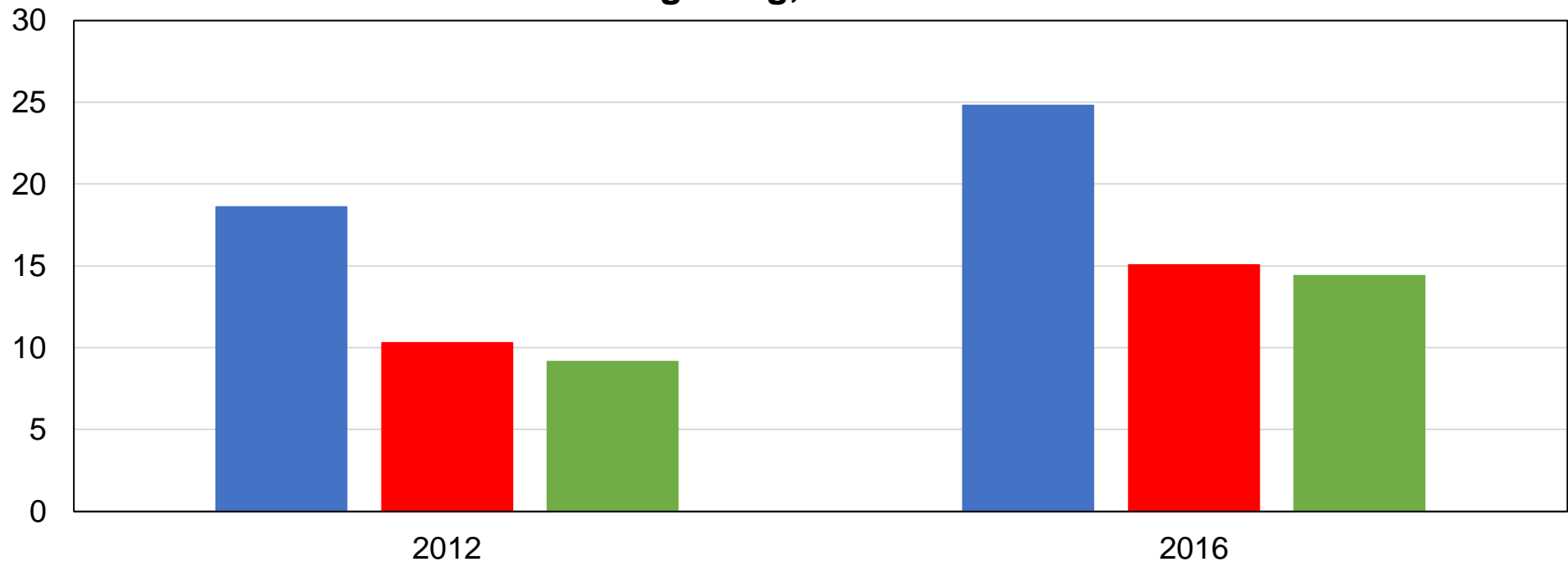
Graphique 13.14 - Le clivage natifs-continentaux à Hong Kong, 2012-2016
