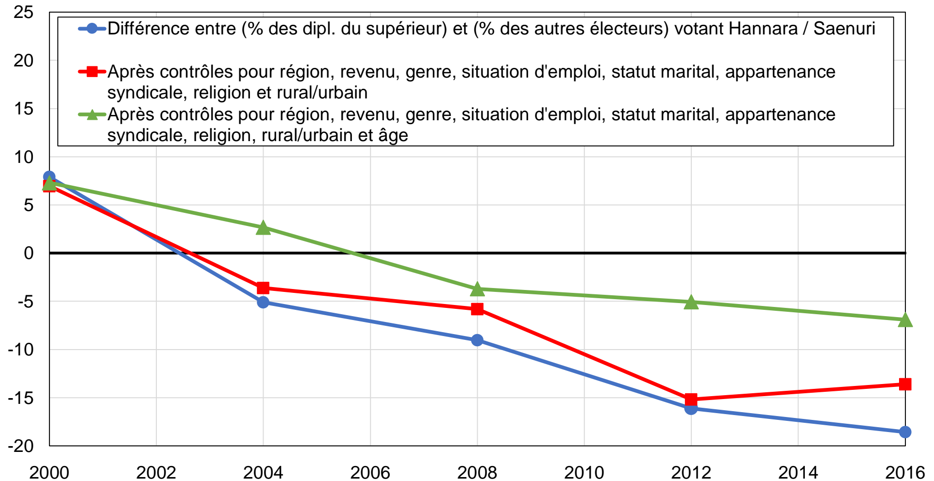
Graphique 13.4 - Le clivage éducatif en Corée du Sud, 2000-2016
